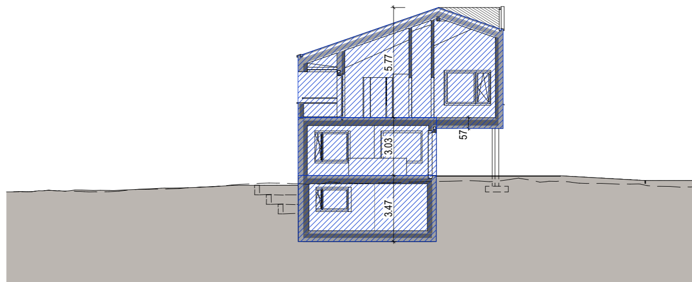
Schnitt B-B
