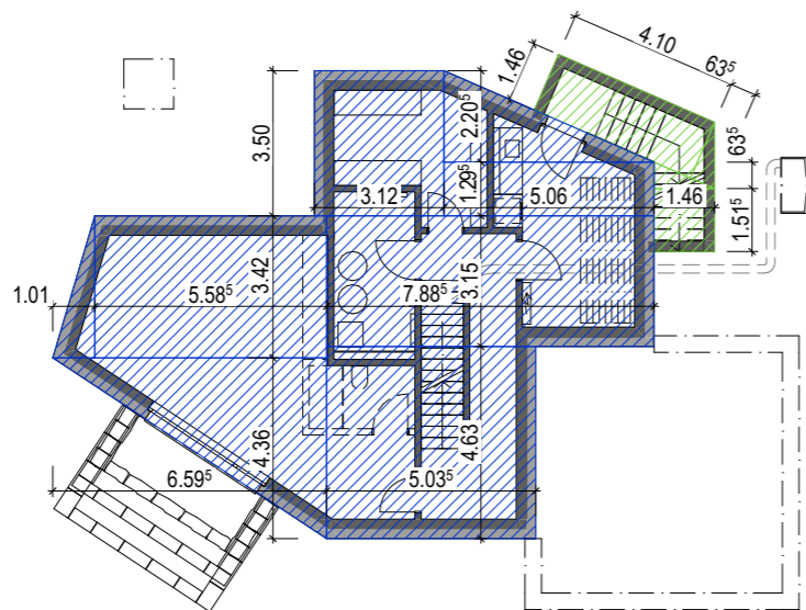
Erdgeschoss
