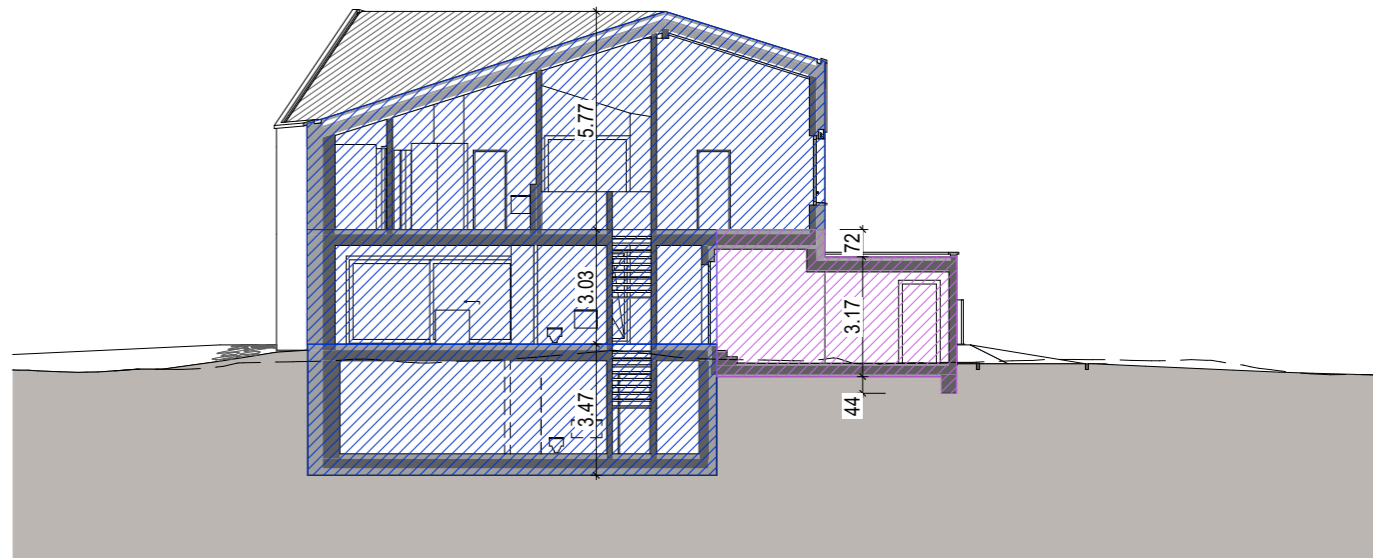
Schnitt A-A
